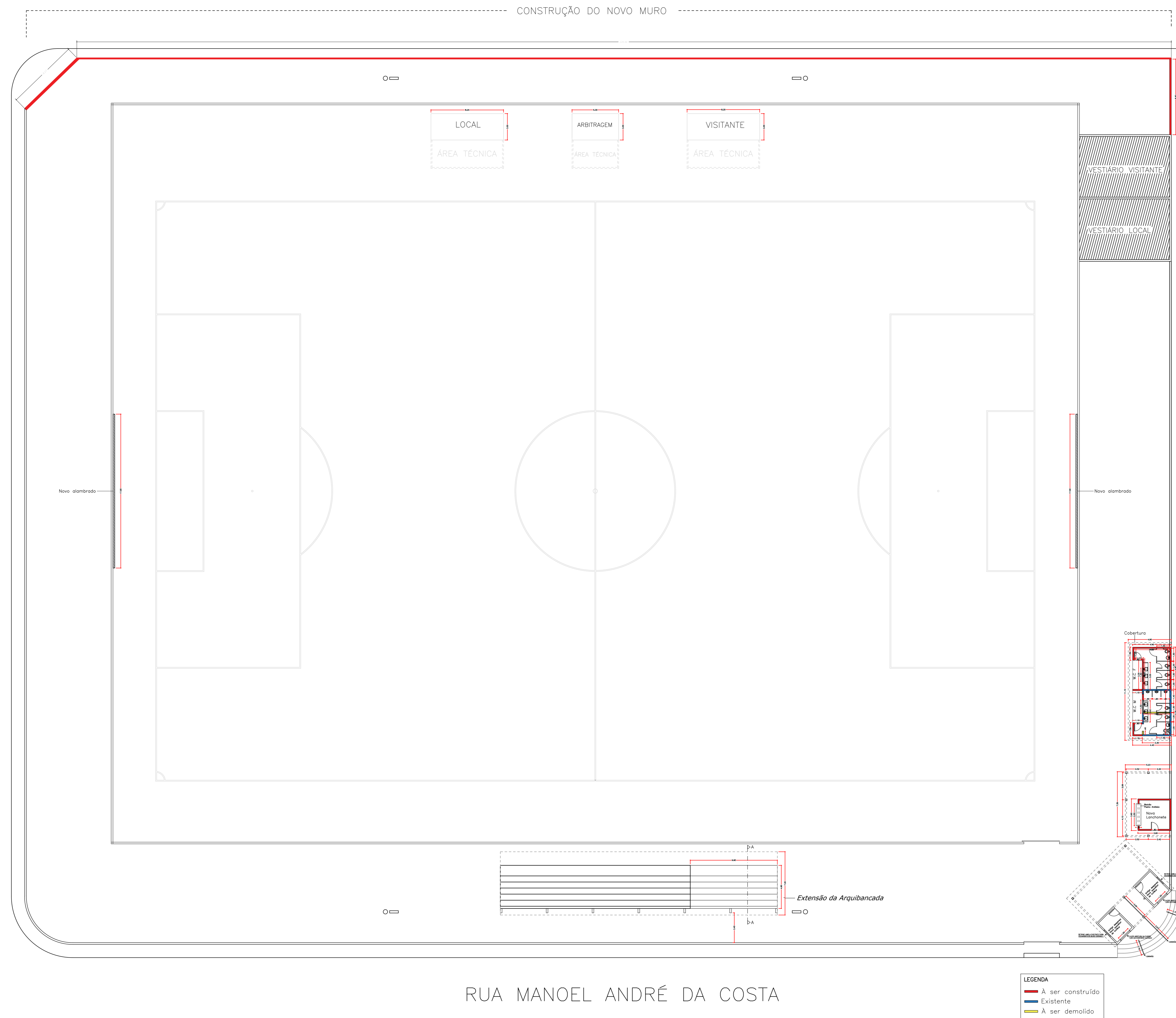
PLANTA DO ESTÁDIO ESC: 1.200
